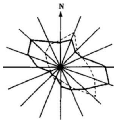
图 2.4.6 结合风象玫瑰图标绘的指北针
